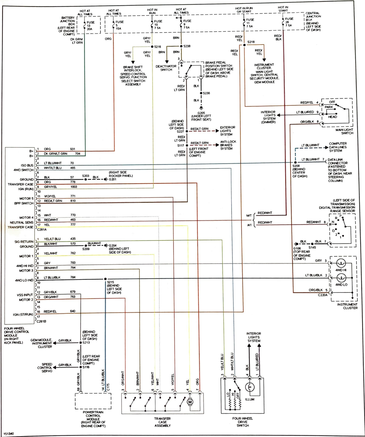
Fig. 60: 4WD Circuit
